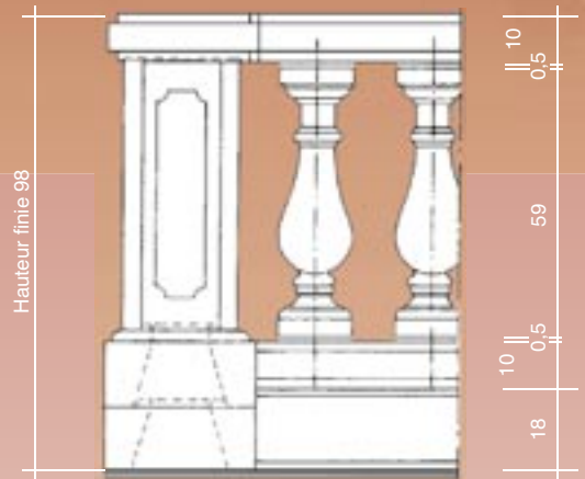
Balustrades posées en garde corps (hauteur finie 98 cm) conformément à la norme NF P 01-012.
